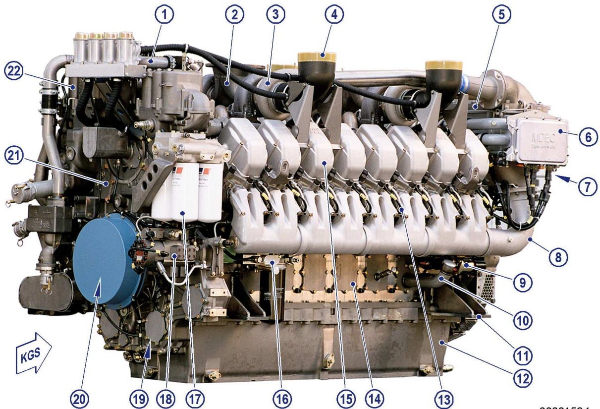
4χρονος κινητήρας MTU 16V 4000, Ισχύος 1390 kW, 1890 HP, 1200 RPM και τα μέρη του
