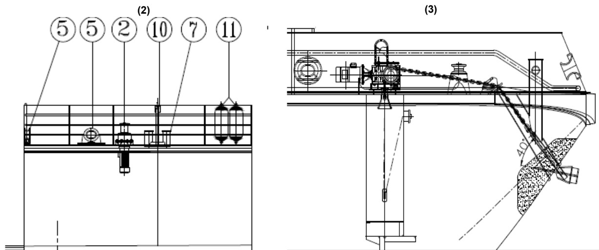
Σκαριφηματική διάταξη μηχανημάτων προσδέσεως πρύμης και μηχανημάτων προσδέσεως / αγκυροβολίας πλώρης
