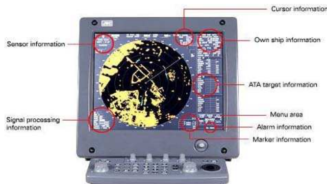
Πληροφορίες που παρέχει η συσκευή Ραντάρ με ενσωματωμένο το σύστημα ARPA
