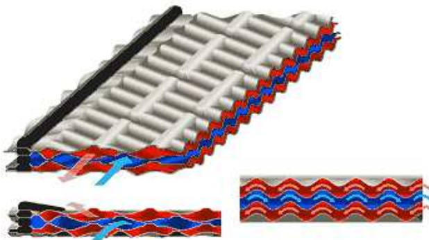
Αυλακώσεις μεταξύ πλακών όπου με κόκκινο χρώμα είναι το ψυχώμενο υγρό και με μπλε είναι το μέσο ψύξης ενός πλακοειδή εναλλάκτη και στις άκρες με μαύρο οι φλάντζες στεγανοποίησης
