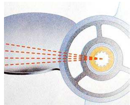
Το «κουπάρισμα» κατά μήκος της γραμμής του rake, μεταβάλλει το rake
