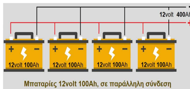
Μπαταρίες 12volt 100Ah, σε παράλληλη σύνδεση Συστοιχία συσσωρευτών σε παράλληλη σύνδεση (4X100Ah) 400Ah 12Volt
