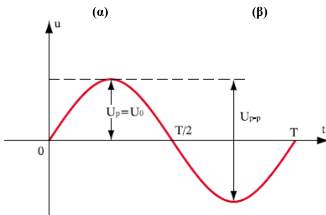
Σχήμα: (α) την τιμή κορυφής ( U_p=U_0 )(β) την τιμή από κορυφή σε κορυφή ( U_{p-p} )
