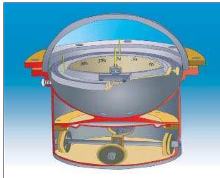
Μηχανισμός Γυροπυξίδας
