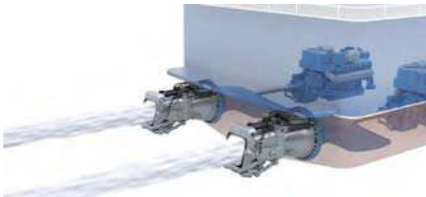
Σύστημα προωθητήρων αντίδρασης Rolls-Royce KAMEWA σε σκάφος
