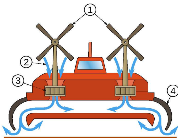
Σχηματική παράσταση πρόωσης Α/Σ. 1. Έλικες 2. Ρεύμα αέρος, 3. Ανεμιστήρες, 4. Πλαστική περίζωση αέρος κοινώς φούστα Ακίνητοποιημένο επιπλέει στον πλωτήρα στον οποίο στηρίζεται
