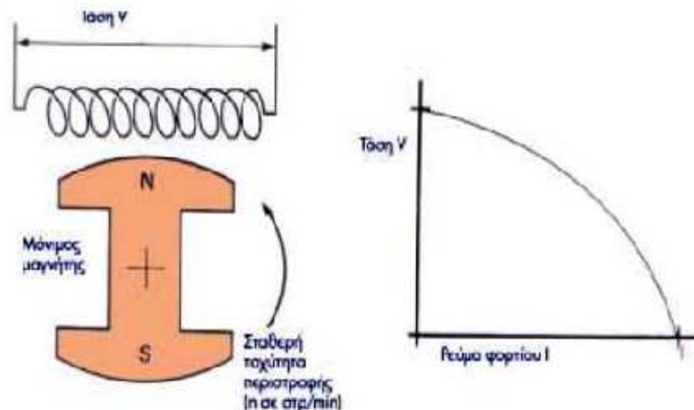
Γεννήτρια με διέγερση μόνιμου μαγνήτη η χαρακτηριστική φορτίου της
