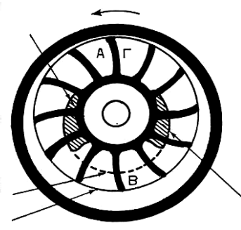
Με εκκεντρικό κυκλικό κέλυφος (plate pump) & με ελλειπτικό κέλυφος
