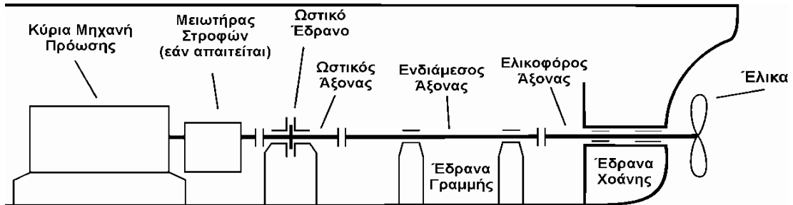
Μέρη πρόωσης του σκάφους: 1. Κινητήρια μηχανή, 2. Μειωτήρας στροφών (εάν απαιτείται), 3. Ωστικό έδρανο, 4. Ωστικός άξονας (Ωστικός τριβέας), 5. Ενδιάμεσος άξονας (άτρακτος), 6. Έδρανα γραμμής, 7. Ελικοφόρος άξονας (άτρακτος), 8. Έδρανα χοάνης, 9. Έλικα (αφορά μεγάλα σκάφη)
