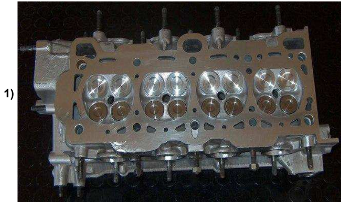
1) Κυλινδροκεφαλή με 4 βαλβίδες, δύο Εισαγωγής και δύο Εξαγωγής ανά κύλινδρο και 2) ο κορμός πετρελαιοκινητήρα
