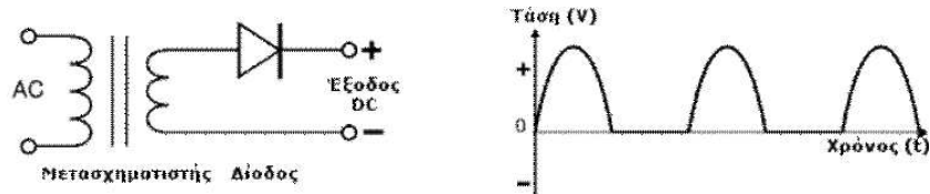
Γραφική παράσταση της μετατροπής της εναλλασσόμενης τάσης (AC) σε συνεχή τάση (έξοδος) (DC)
