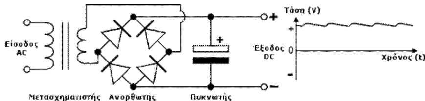
Γραφική παράσταση Μετασχηματιστή+Ανορθωτή+Πυκνωτή
