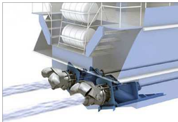
Water jet - Προωθητήρες αντίδρασης
