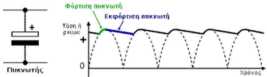
Γραφική παράσταση φόρτισης-εκφόρτισης πυκνωτή
