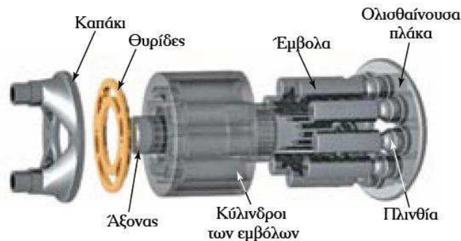
Αντλία με περιστρεφόμενο σώμα κυλίνδρων
