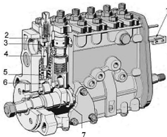
Εμβολοφόρος αντλία Υ.Π για δκύλινδρη πετρελαιομηχανή πετρελαίου 1. Άκρο οδοντωτού κανόνα, 2. Βαλβίδα παροχής, 3. Δίοδος εισόδου καυσίμου, 4. Έμβολο με τομή έλικας, 5. Ελατήριο επαναφοράς, 6. Ωστήριο, 7. Εκκεντροφόρος άξονας
