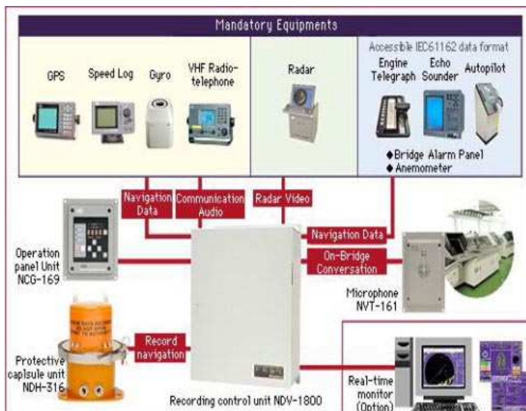
Οι διασυνδέσεις του VDR με άλλα ναυτικά όργανα
