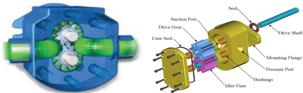
Τομή Γραναζωτής αντλίας και τα μέρη της
