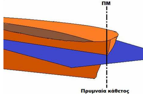
Τρισδιάστατη σχηματική απεικόνιση Πρυμναίας καθέτου
