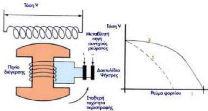
Γεννήτρια με πηνίο διέγερσης και οι χαρακτηριστικές φορτίου με σταθερή ένταση πεδίου (1) και με μεταβολή της έντασης πεδίου (2), για να διατηρήσουμε σταθερή την τάση της γεννήτριας.
