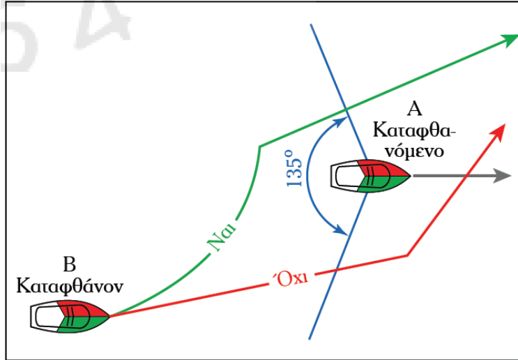
Καταφθάνον πλοίο το οποίο φυλάσσει το καταφθάνομενο και διέρχεται από πρύμα με αποκλίνουσα αναπρώρηση, απομακρυνόμενο προς την επιθυμητή πλευρά
